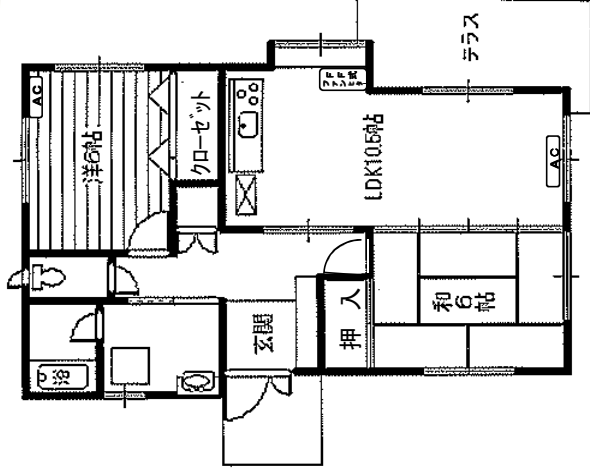
【間取図】
